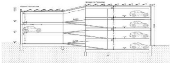
Abbildung 16: Schnitt Parkhaus (GBC) Die Gesamthöhe des Parkhauses beträgt 10,55 m am tiefsten Punkt des Split-Level-Designs (vgl. Abbildung 16). Die lichte Höhe beträgt 2,10 m, die Geschosshöhe beläuft sich auf 2,75 m
