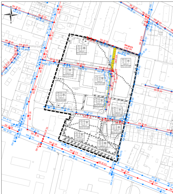
Abbildung 17: Führung der Schutz- und Regenwasserkanäle (Plan genordet, unmaßstäblich)
