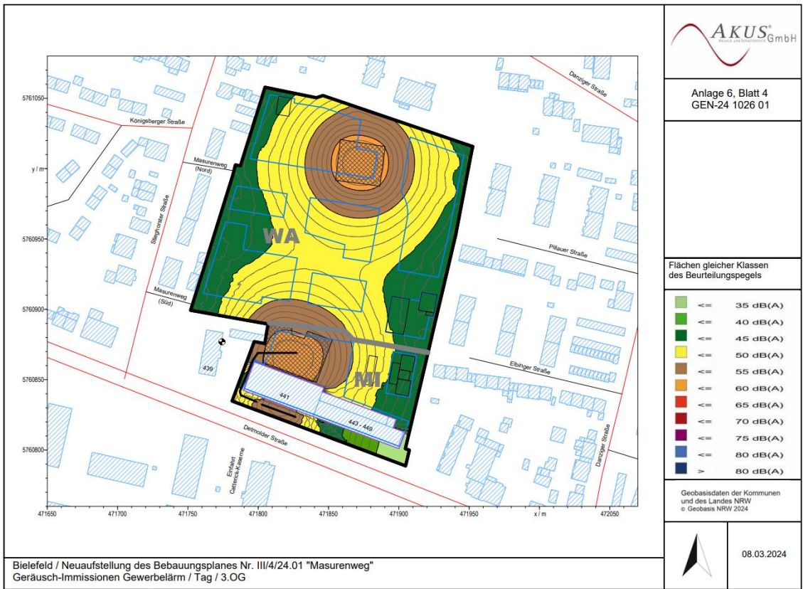
Abbildung 14: Schalltechnische Untersuchung; Geräusch-Immissionen Gewerbelärm am Tag im 3. Obergeschoss Quelle: Akus GmbH, Bielefeld, Anlage 6 Blatt 4 (08.03.2024, Auftragsnummer BLP-24 1026 01)
