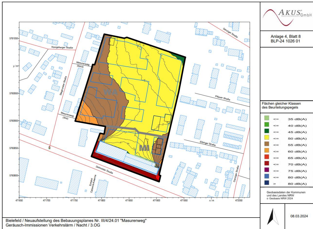
Abbildung 13: Schalltechnische Untersuchung; Verkehrslärm in der Nacht im 3.Obergeschoss
