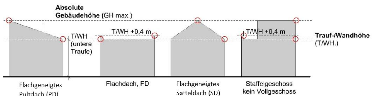
Abbildung 9: Prinzipskizze obere Höhen-Bezugspunkte
