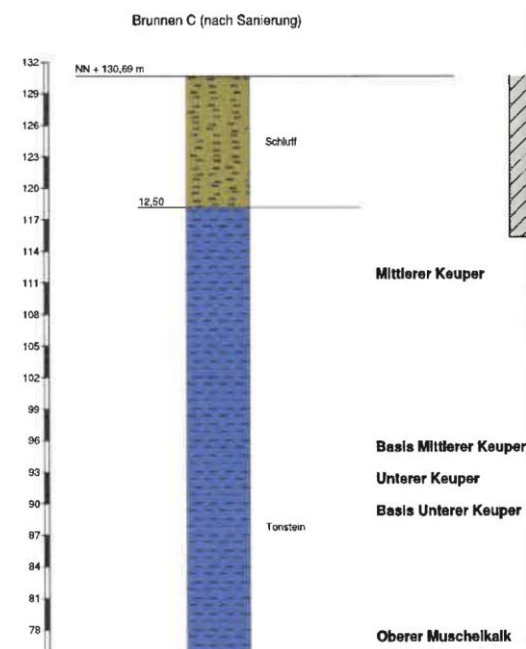
Abbildung 19: Zeichnerische Darstellung des Bohrprofils nach DIN 4023 (Oberflächennaher Ausschnitt), Ing.-Büro ENVITEC GmbH, 10.01.2017
