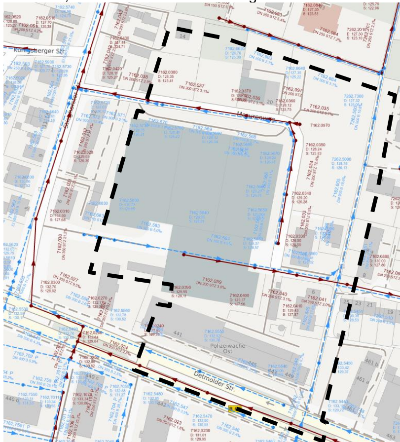
Abbildung 16: Kanalbestand (genordet, unmaßstäblich)
