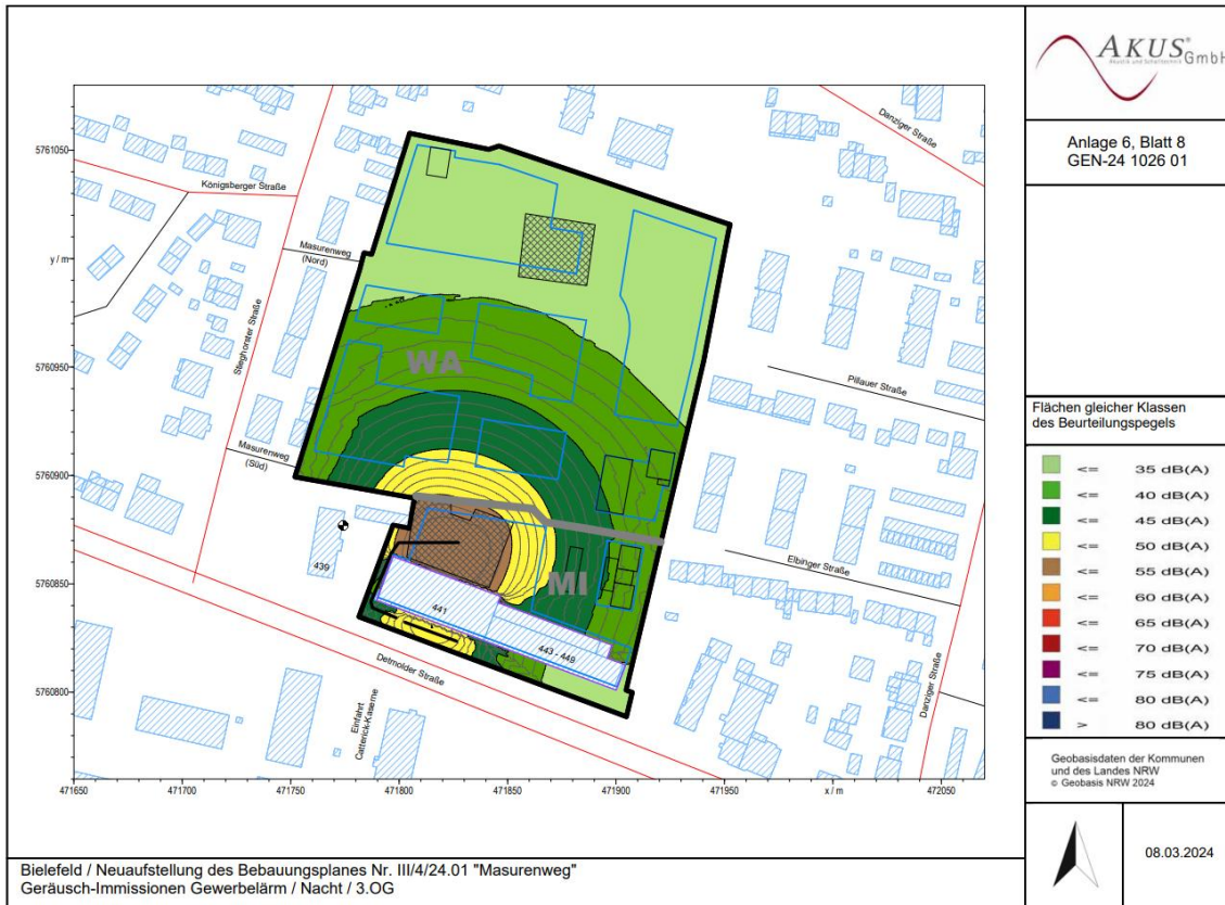
Abbildung 15: Schalltechnische Untersuchung; Geräusch-Immissionen Gewerbelärm in der Nacht im 3. Obergeschoss Quelle: Akus GmbH, Bielefeld, Anlage 6 Blatt 8 (08.03.2024, Auftragsnummer BLP-24 1026 01)
