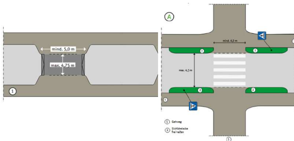
Abbildung 86: Vorgezogener Seitenraum mit Aufpflasterung (links) | Fußgängerüberweg mit Begrünung (rechts) (Quelle: Musterlösungen Knotenpunktgestaltung (AGFS NRW))
