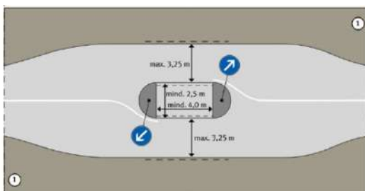
Abbildung 78: Mittelinsel mit beidseitigem Fahrbahnversatz (Quelle: AGFS Leitfaden Querungsstellen Fußverkehr) (links) | Baumbeste zur Verkehrsberuhigung (Quelle: www.stvo2go.de ) (rechts)
