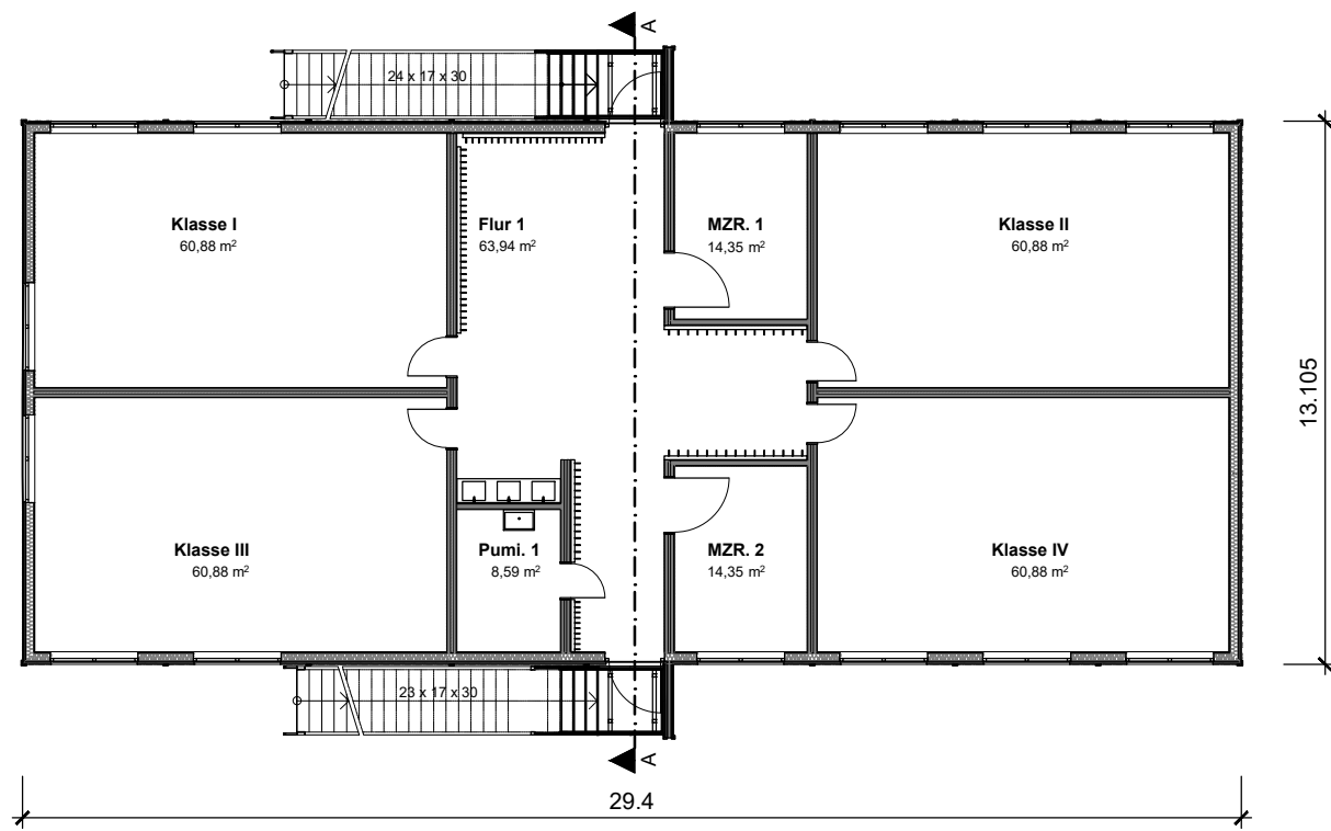
GRUNDRISS ERDGESCHOSS
