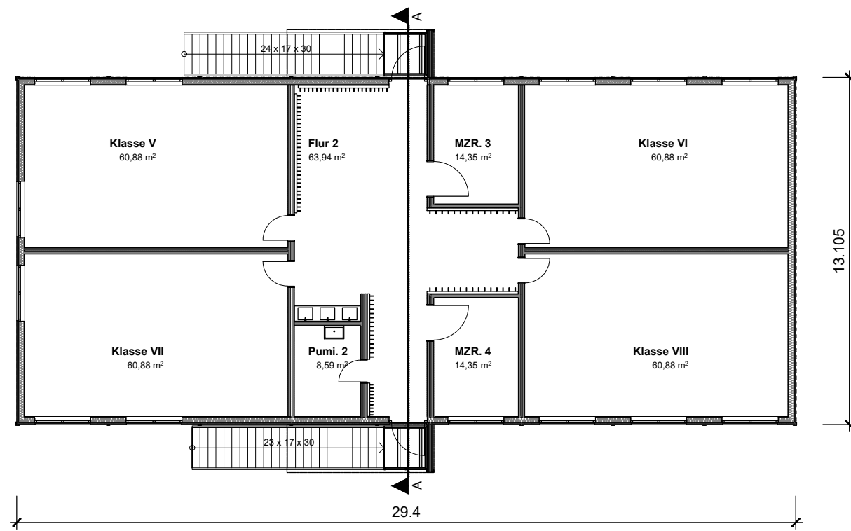
GRUNDRISS OBERGESCHOSS
