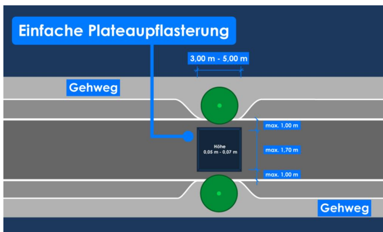
Abbildung 7: Einfache Plateauaufpflasterung (Quelle: www.stvo2go.de )
