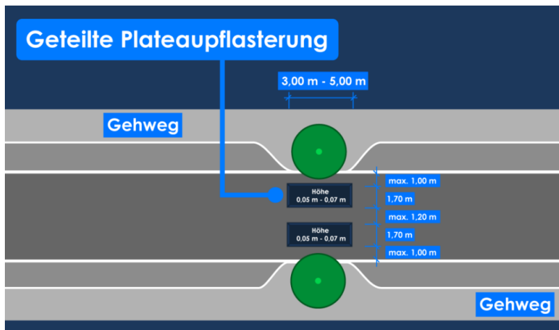
Abbildung 6: Geteilte Plateauaufpflasterung (Quelle: www.stvo2go.de )
