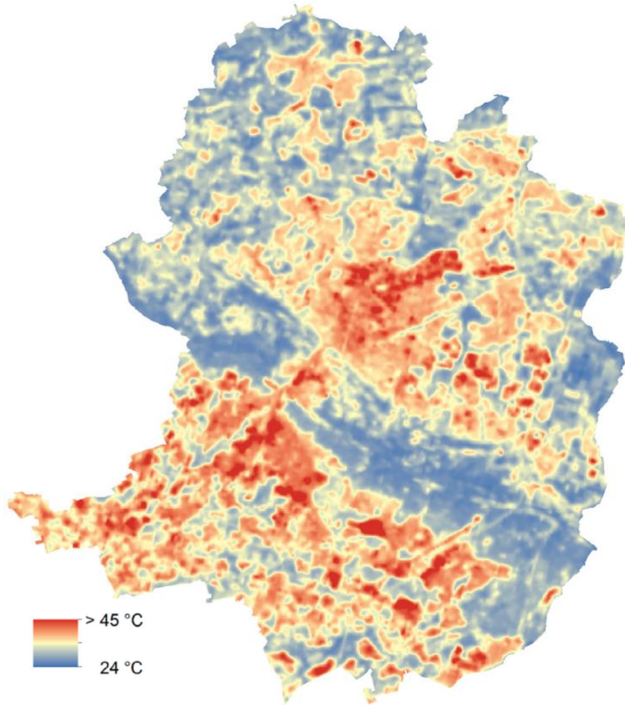
Mittlere Oberflächentemperatur in °C an einem warmen Sommertag zwischen Juni-August 2019 aus LANDSAT-Satellitendaten (LUP 2020)
