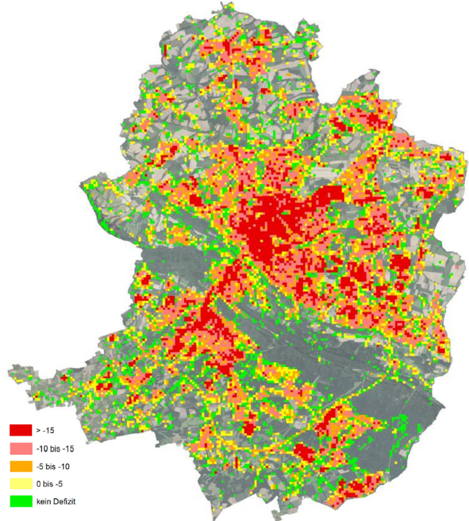
Fehlendes Grünvolumen in \text{m}^3/\text{m}^2 zur Beschränkung der Oberflächentemperatur auf 31 °C. Berechnung aus Satelliten- und Luftbilddaten (LUP 2020)
