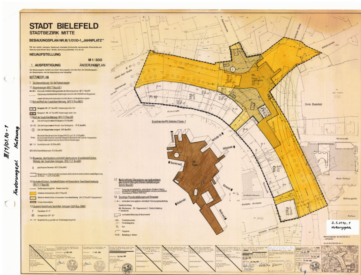
Nutzungsplan des Bebauungsplans Nr. III/1/01.10-1 „Jahnplatz“
