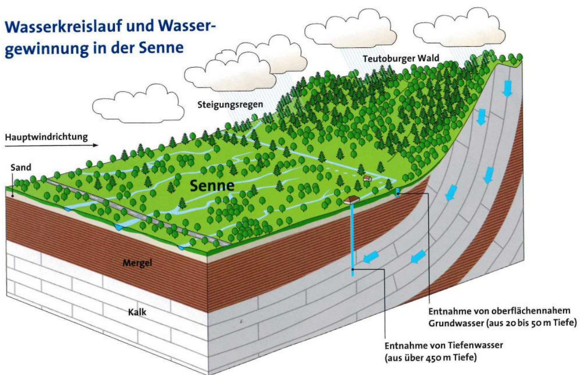
Abbildung 14 Blockbild Senneförderung, Auszug aus „Trinkwasser für Bielefeld“ (Quelle: Eigenpublikation SWB, 2012)
