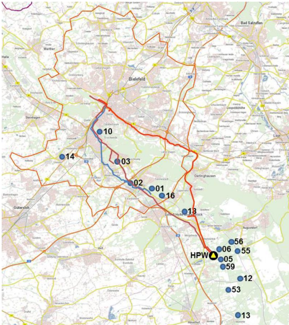
Abbildung 10 Lageplan Wasserwerke, Zubringerleitungen (rot, braun und blau) und Hauptpumpwerk (HPW) (Quelle: SWB, 2017)
