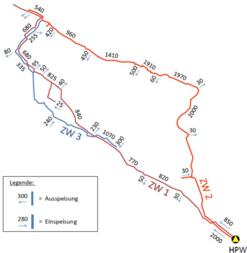
Abbildung 13 Transportnetz vom Hauptpumpwerk (HPW) in Stukenbrock ins Stadtgebiet Bielefeld mit lokalen Ein- und Ausspeisungen in \text{m}^3/\text{h} (Quelle: SWB, 2017)
