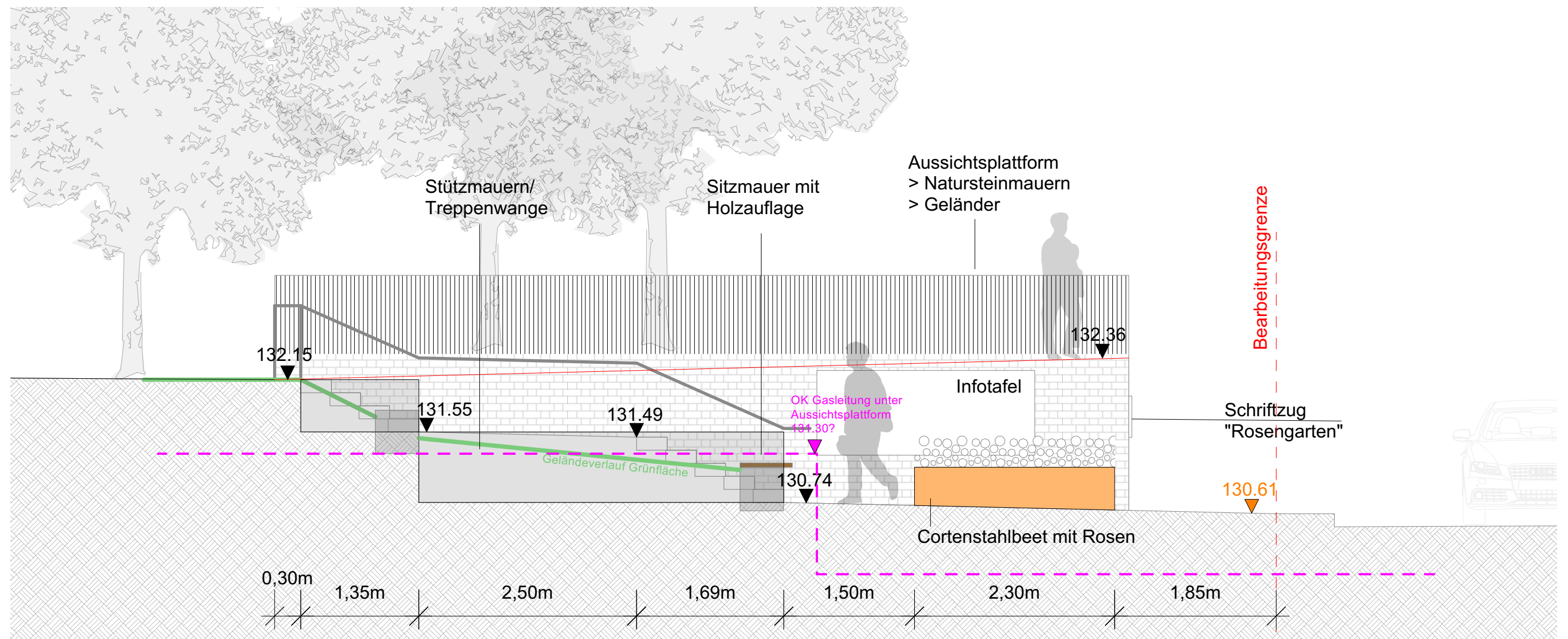
Schnittansicht Aussichtsplattform Haupteingang, M 1:50
