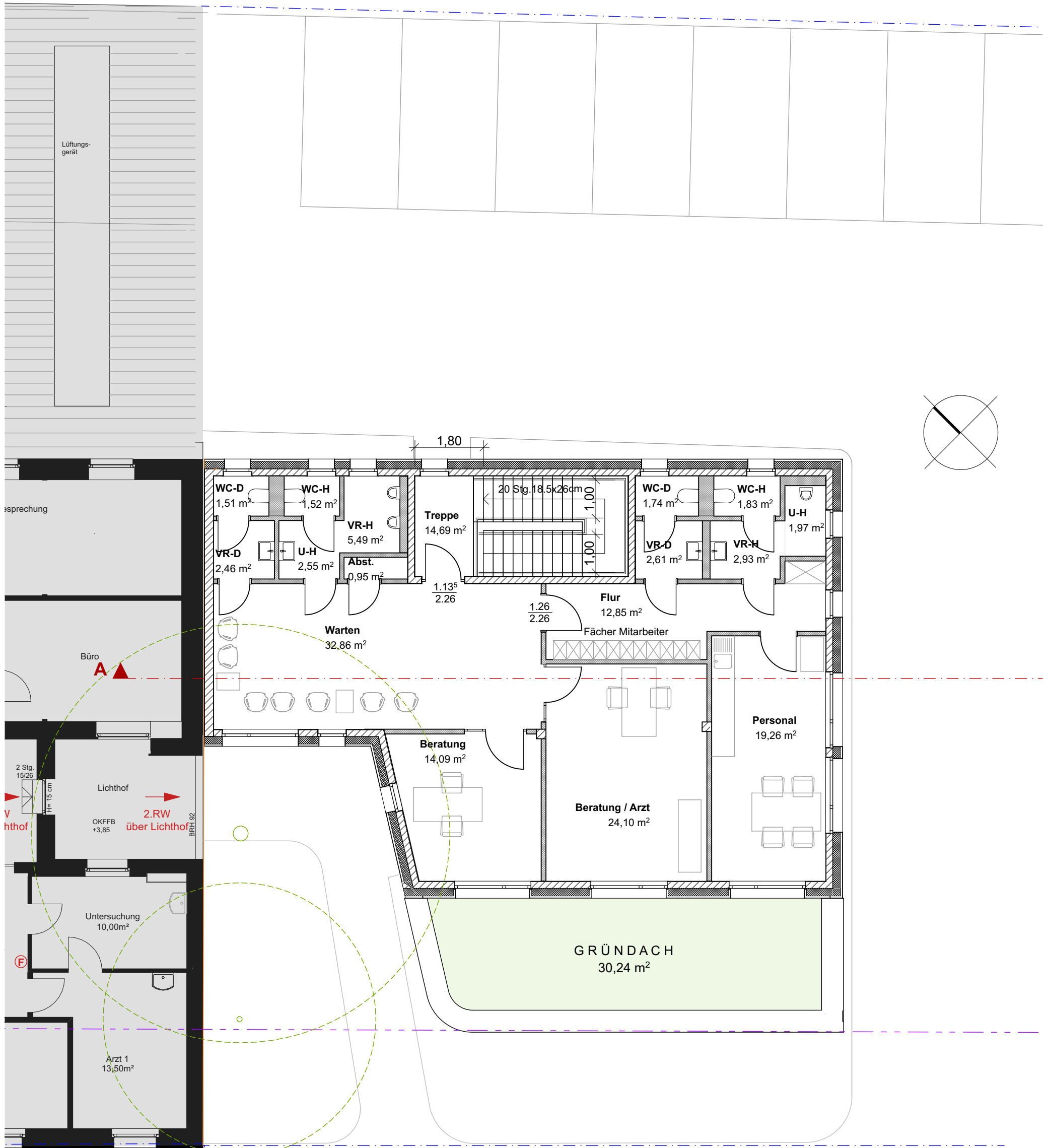
GRUNDRISS 1.OBERGESCHOSS 1:100
