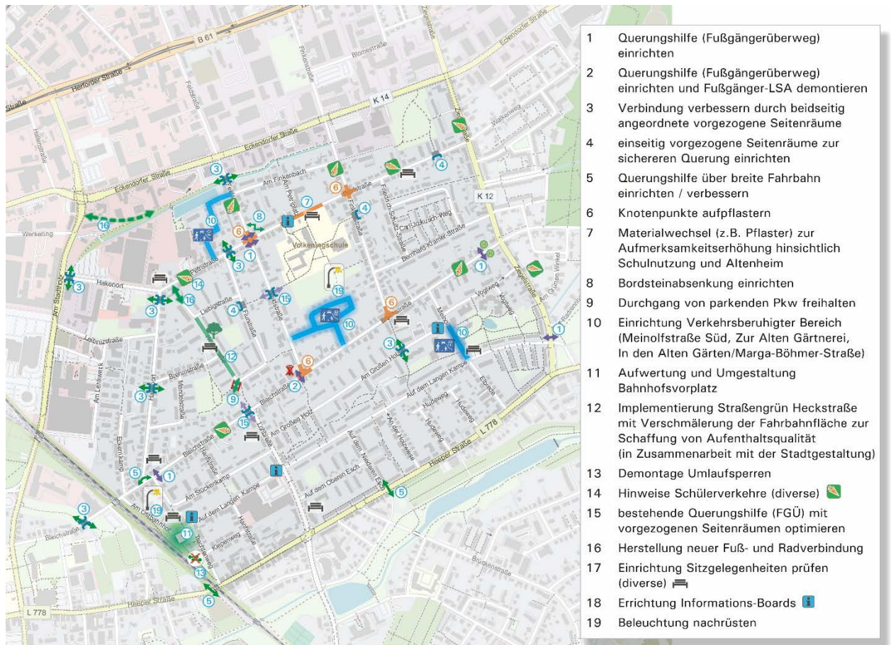
Abb. 40 Maßnahmenkonzept Fußverkehr
