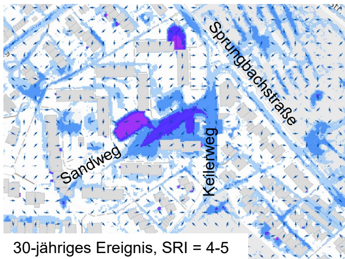
Abbildung 2: Überflutungen bei unterschiedlichen Starkregenereignissen im Bereich Sprungbachstraße und Keilerweg
