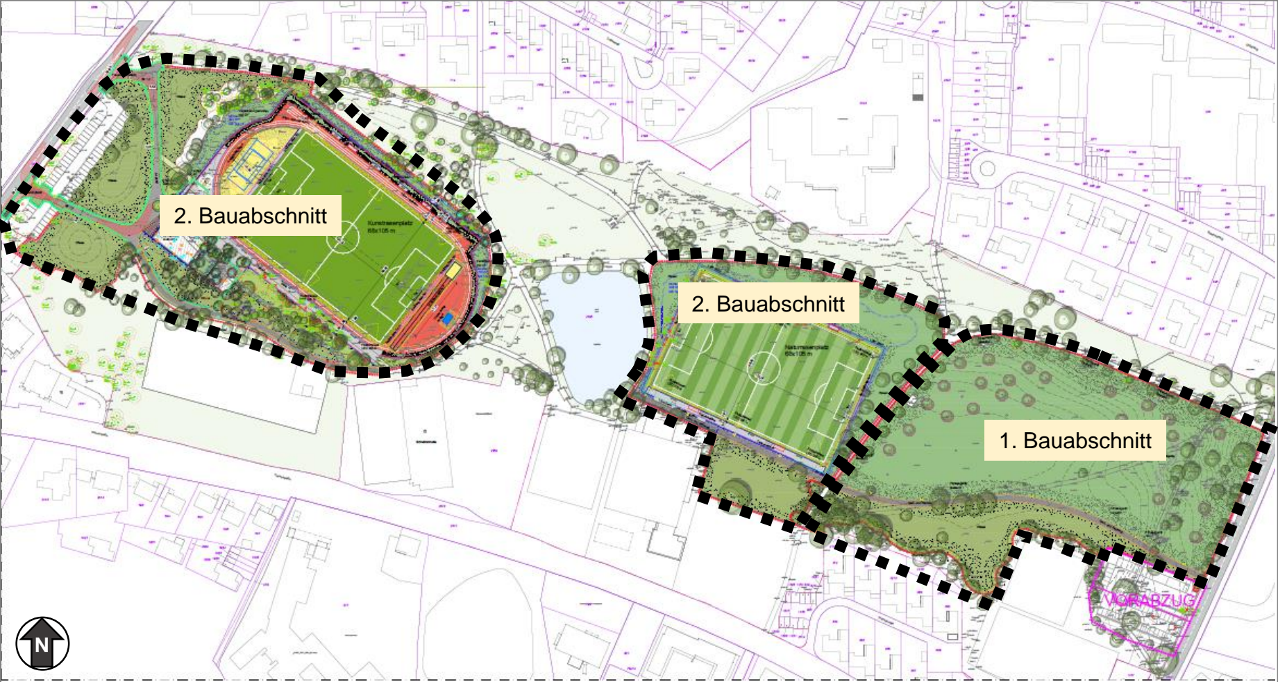
Anlage 1: Lageplan Bauabschnitte
