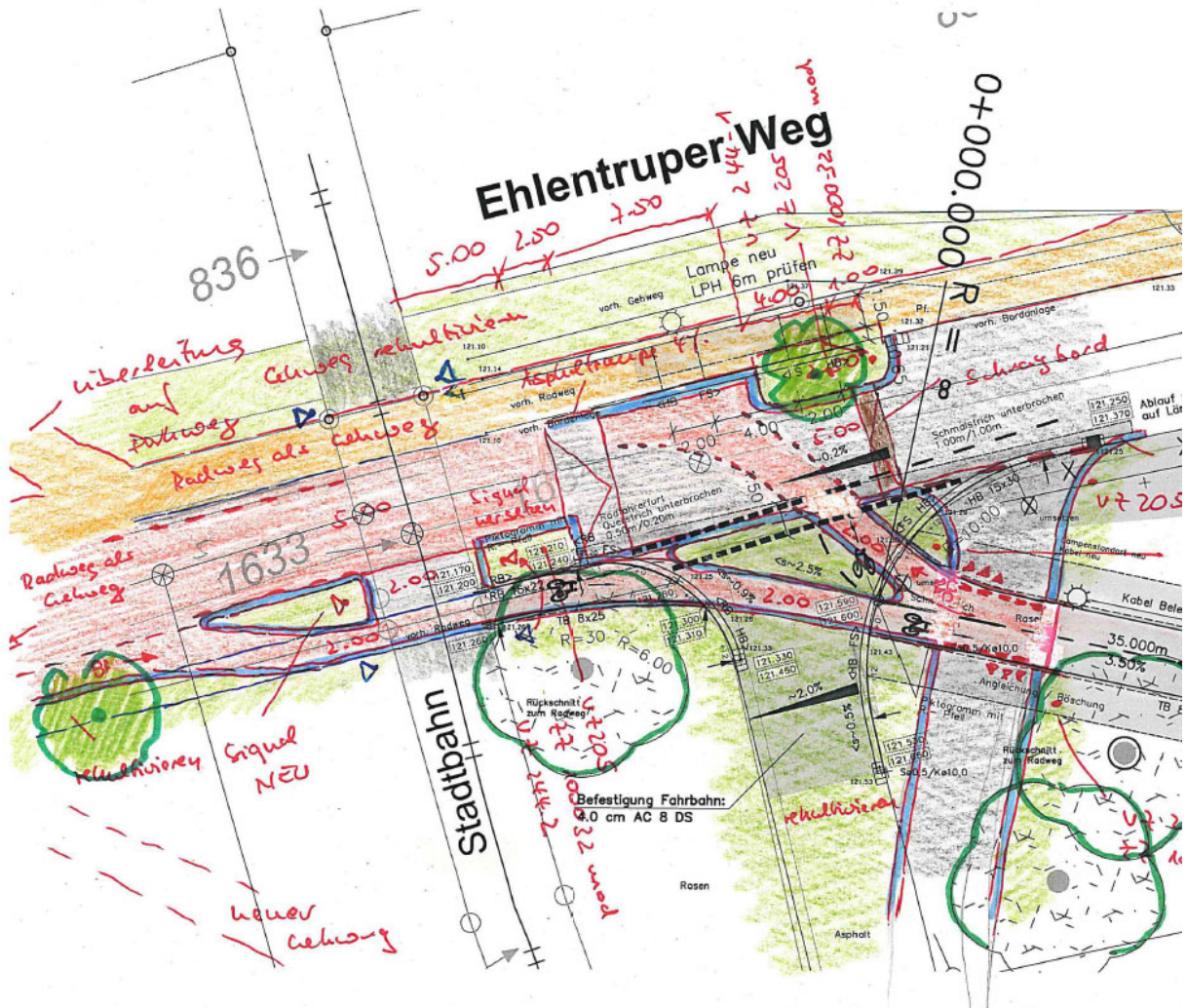
Übergang Fahrradstraße Ehletruper Weg auf Radweg auf Höhe Otto-Brenner-Straße
