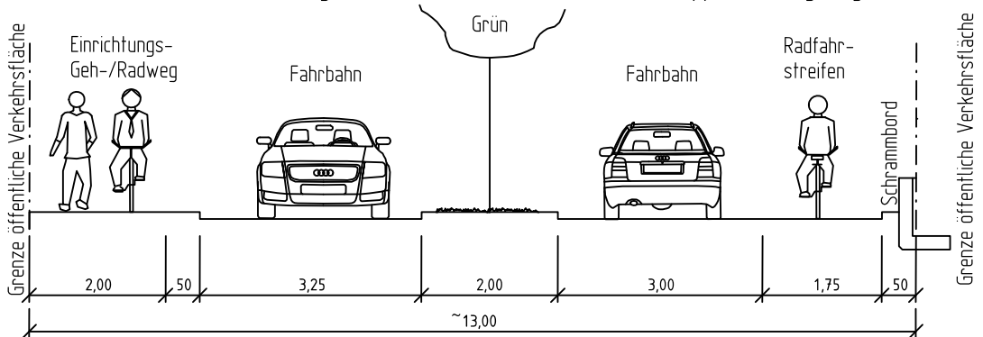
Variante III - Geh- und Radweg West, Radfahrstreifen Ost - Höhe Lipper Hellweg (Engstelle)
