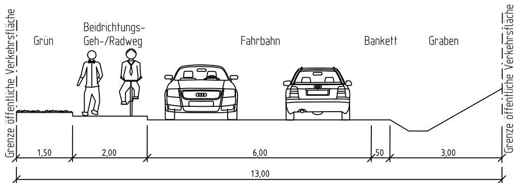
Bestand - Höhe Lipper Hellweg (Engstelle)
