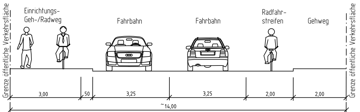
Variante III - Geh- und Radweg West, Radfahrstreifen Ost - Höhe Hausnummer 34
