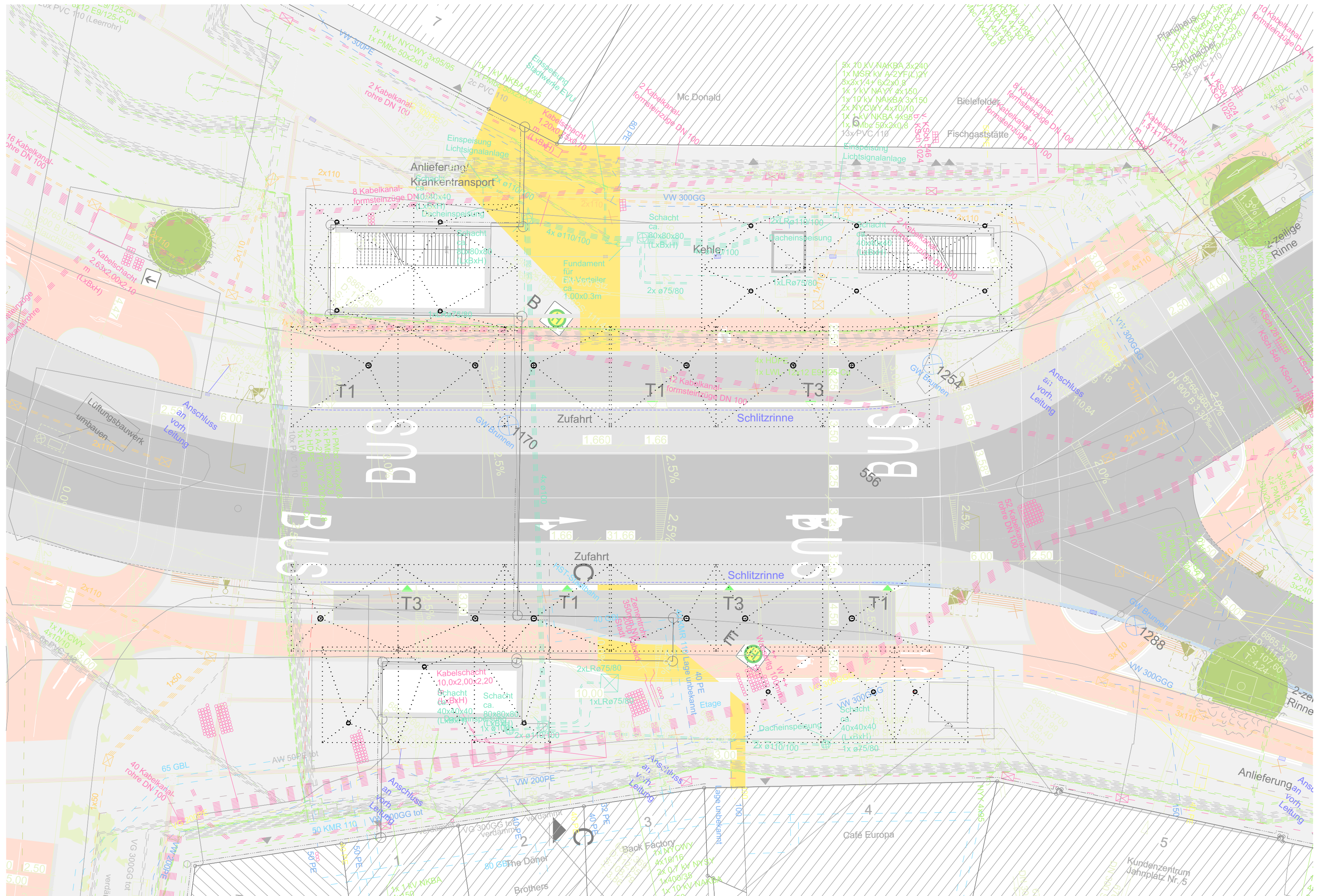
Grundriss
