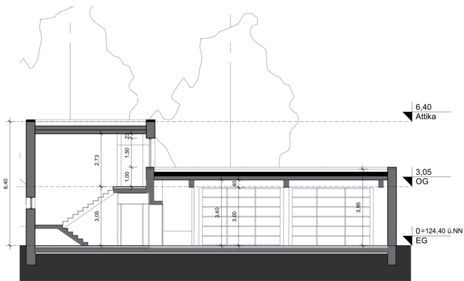
Schnitt B-B
