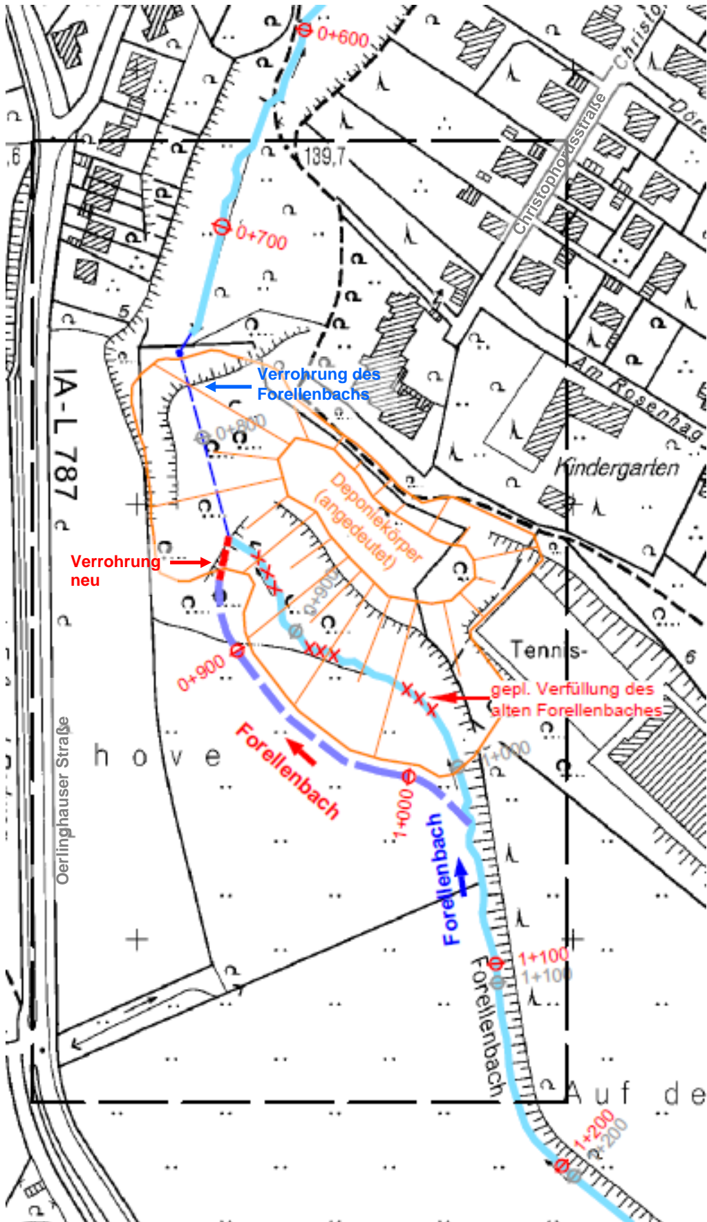
Übersichtsplan Sicherung Deponie 27 Christophorusstraße
