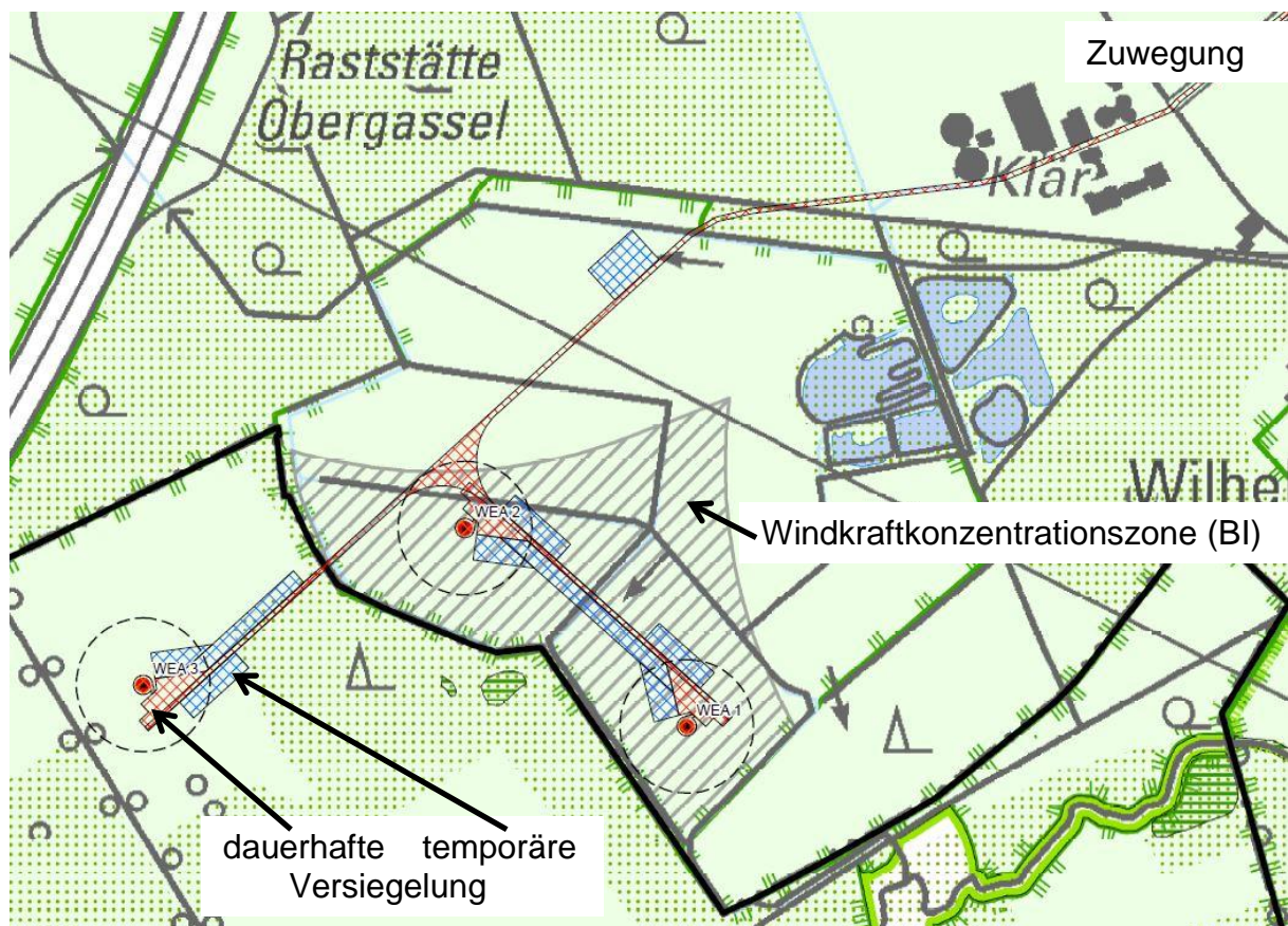
Lageplan
