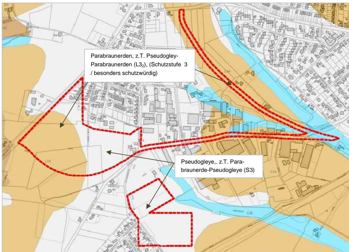
Abb. 4 Darstellungen der Bodenkarte (GLD NRW 2003) mit Abgrenzung des Änderungsbereichs (nicht detailgenau)
