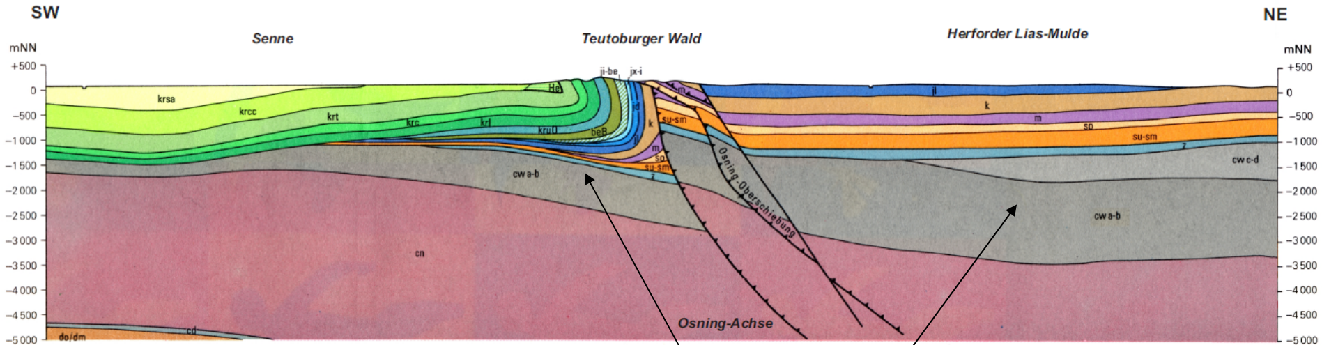
Das Profil soll zur Veranschaulichung der geologischen Lagerungsverhältnisse dienen. Der in der Karte dargestellte Profilverlauf entspricht nicht exakt dem des dargestellten Profils. Die Abfolge der Schichten ist aber vergleichbar. Quelle des Profils: Geologisches Landesamt NRW, Geologische Karte Blatt C3914 Bielefeld, von D. Deutloff, H. Kühn-Velten, G. Michel
