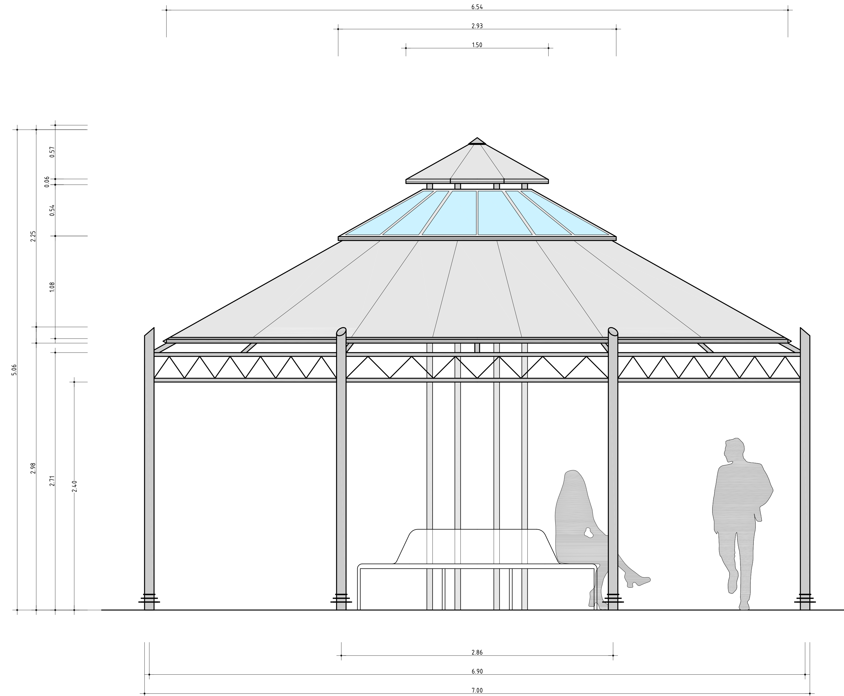
PAVILLON ANSICHT
