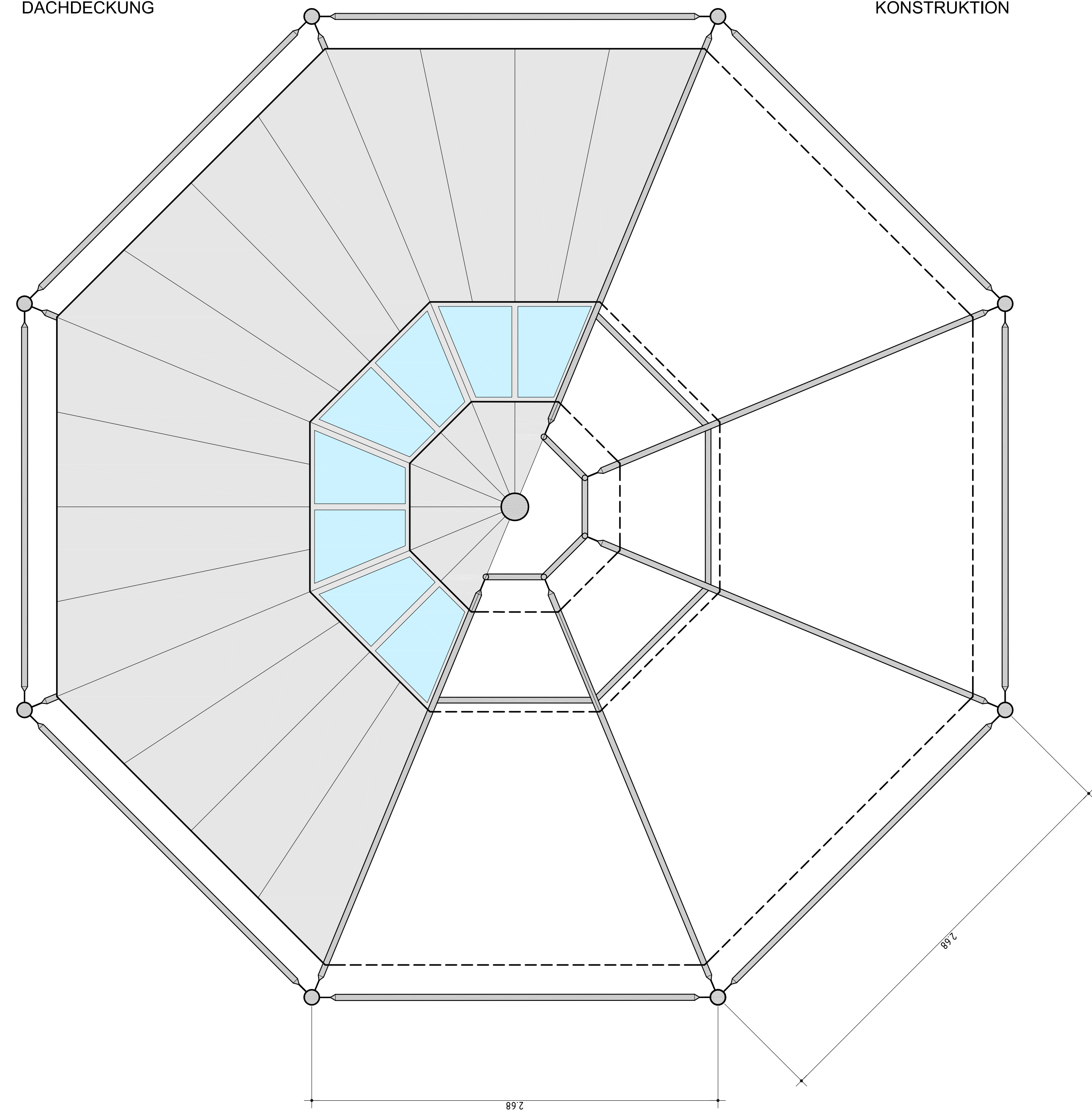
PAVILLON AUFSICHT
