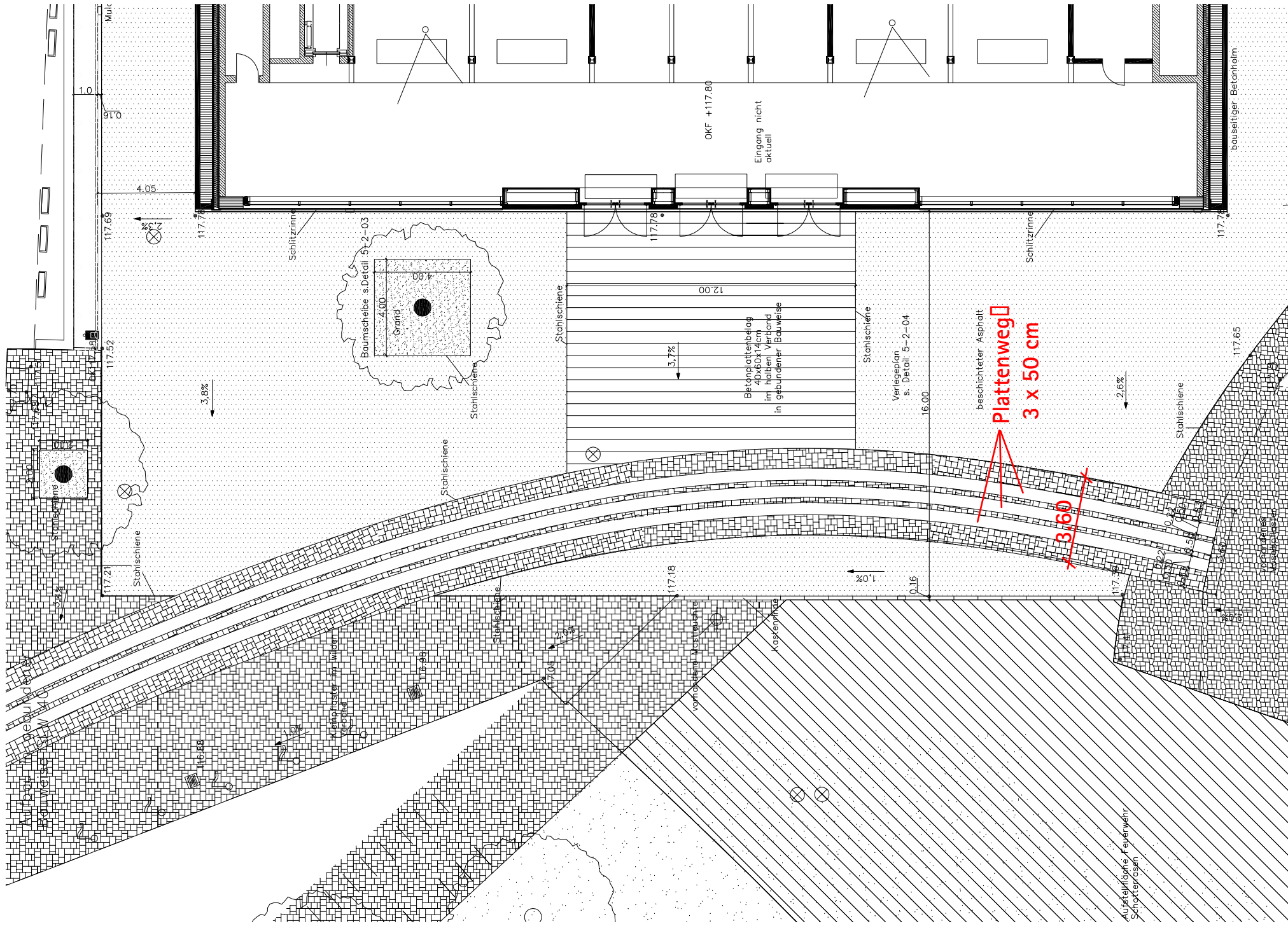
Ausschnitt Aussenanlagen 1:200
